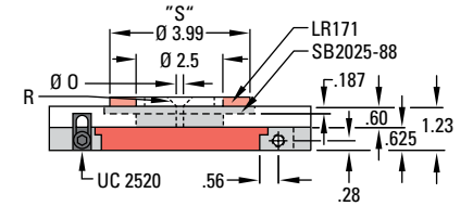
UF 321 Frame Upper – Side View
