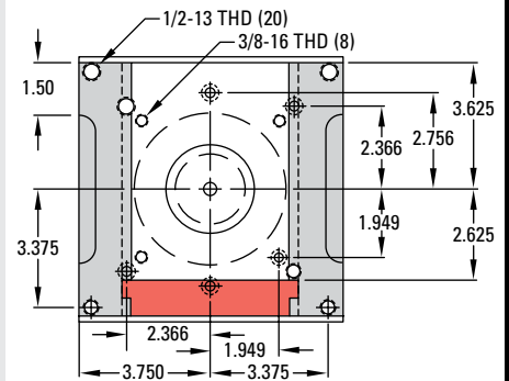
UF 321 Frame Upper – Top View
