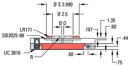
UF 321 Frame Upper – Top View
