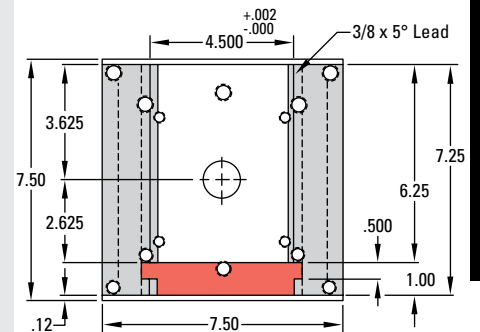
UF 321 Frame Lower – Top View
