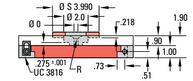
UF 321 Frame Upper – Top View
